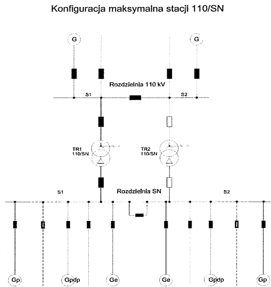
Rys.1. Konfiguracja maksymalna GPZ/RPZ
