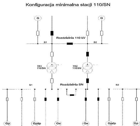
Rys.2. Konfiguracja minimalna GPZ/RPZ
